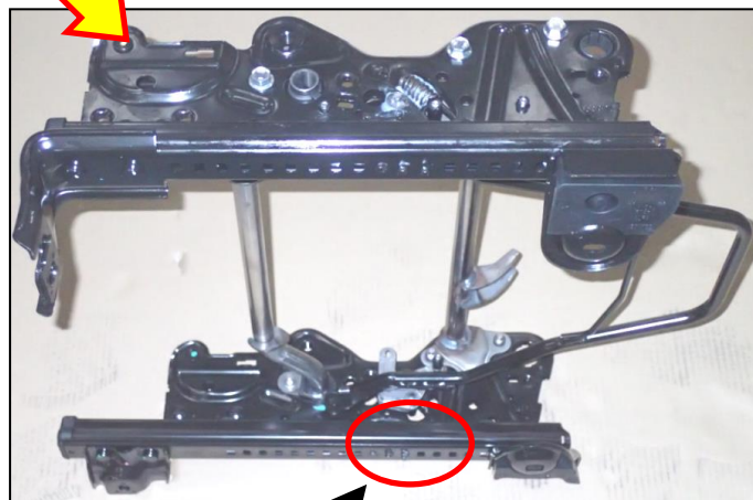
ベースフレームのシートレール (前席右側座席)
